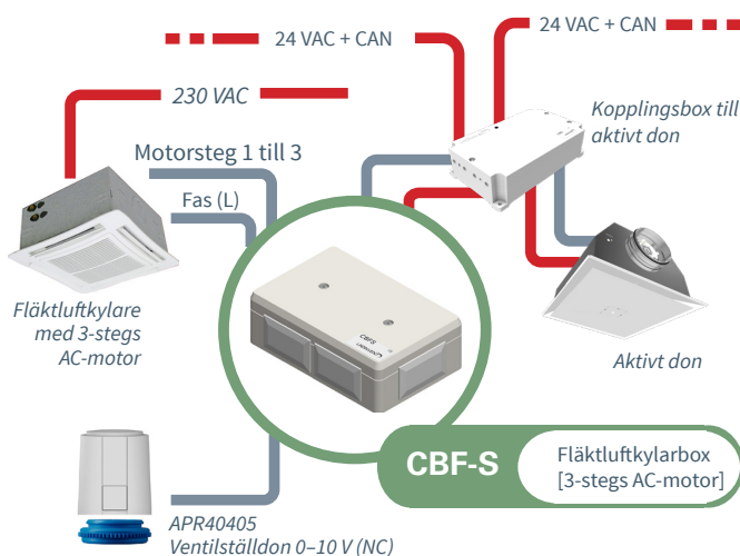
Anslutningsschema CBF-S.
